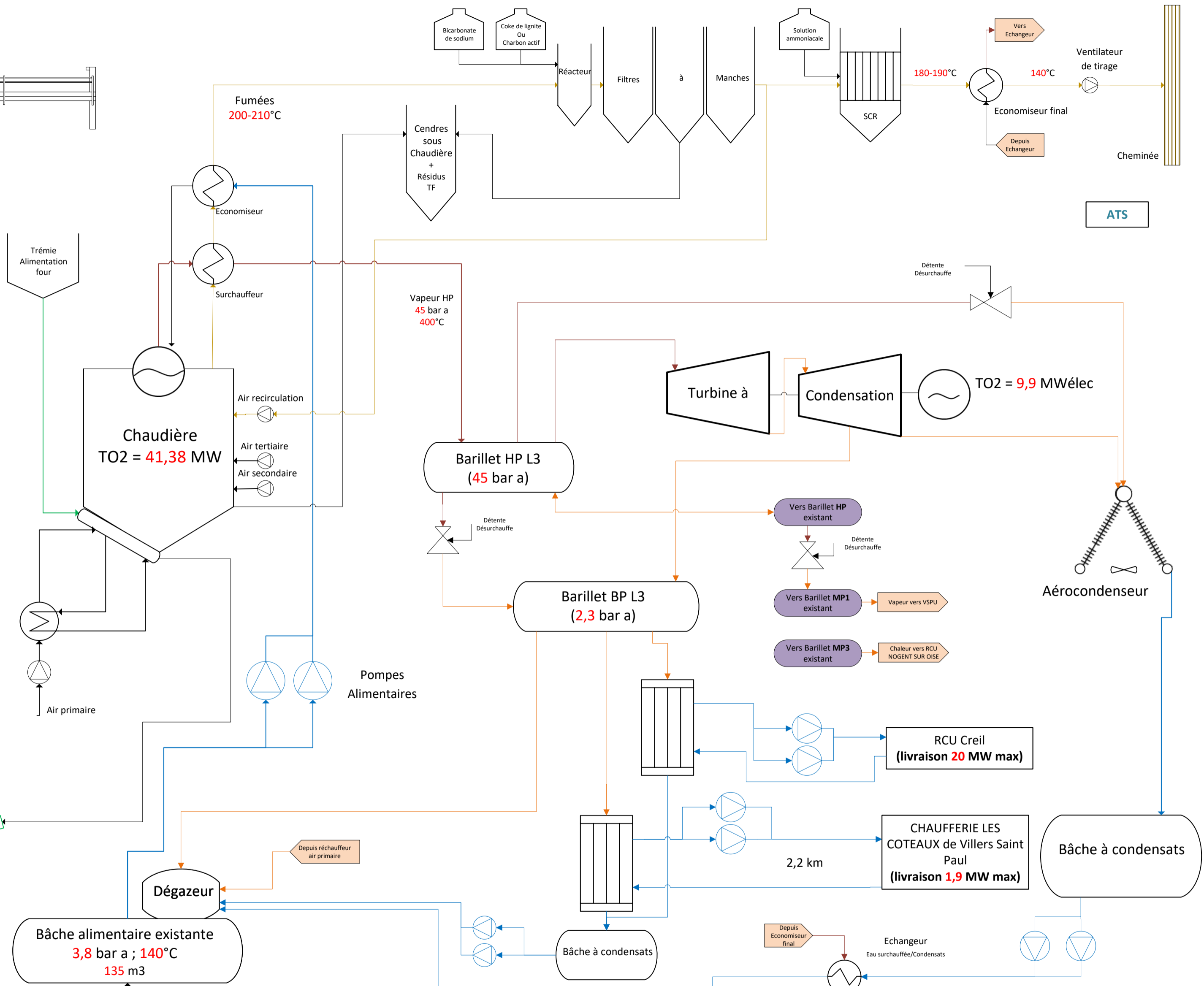
Process Flow Diagram Général Tranche Optionnelle 2
